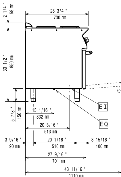
Oldalnézet
